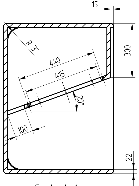
Corte A-A
